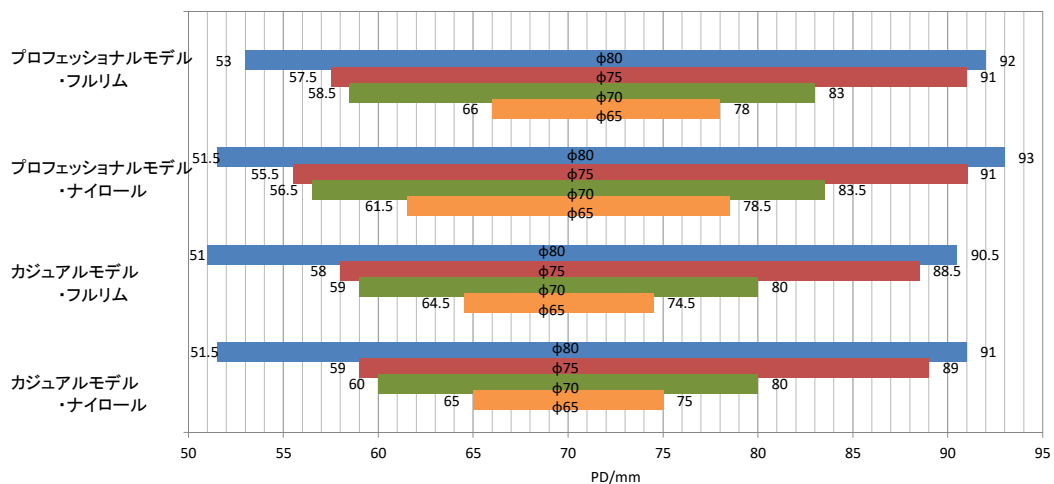
レンズ径別PD有効範囲
