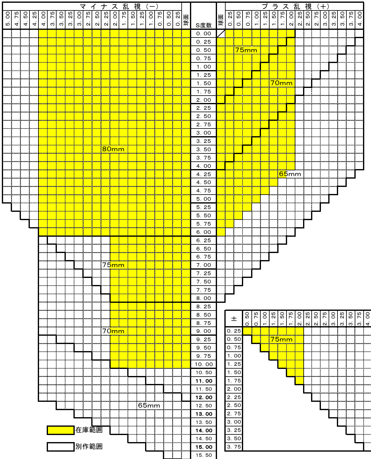
レンズ径別PD有効範囲
